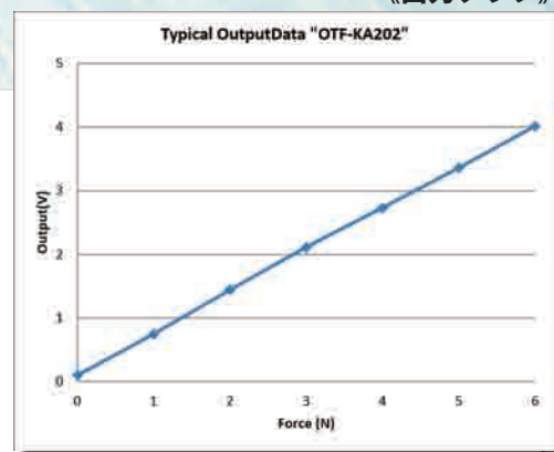
《出力グラフ》
